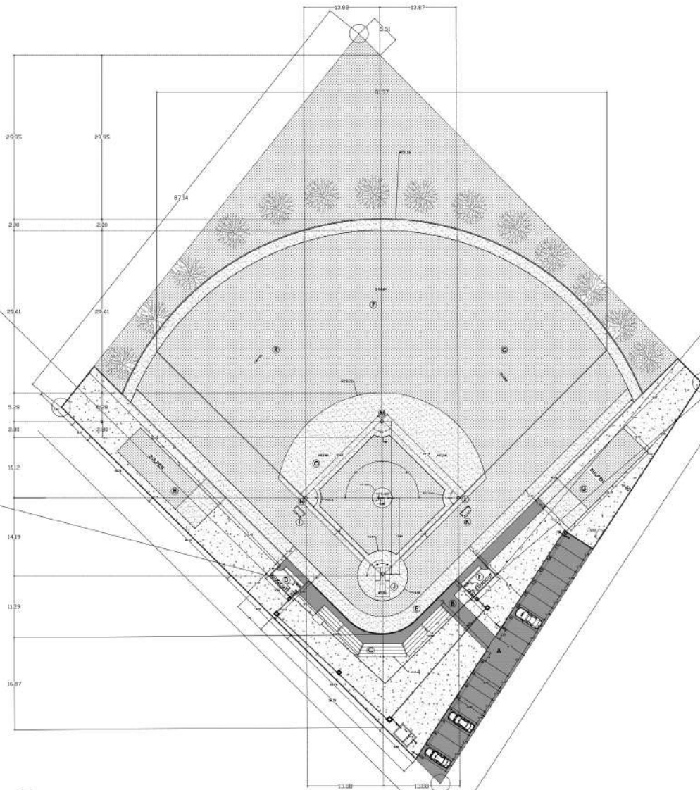
4 PLANTA ARQUITECTONICA DE CONJUNTO A-03 ESC: 1:300
