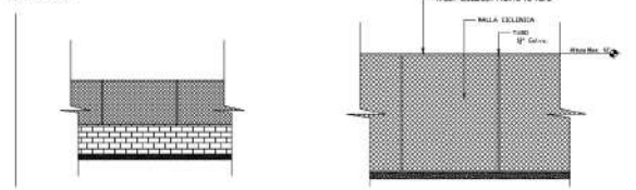
4 VERJA CICLONICA AREA DE HOME A-02 ESC: S/E
