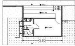
4 SUMINISTRO DE AGUA A-03 DUGOUT ESC: 1:100
