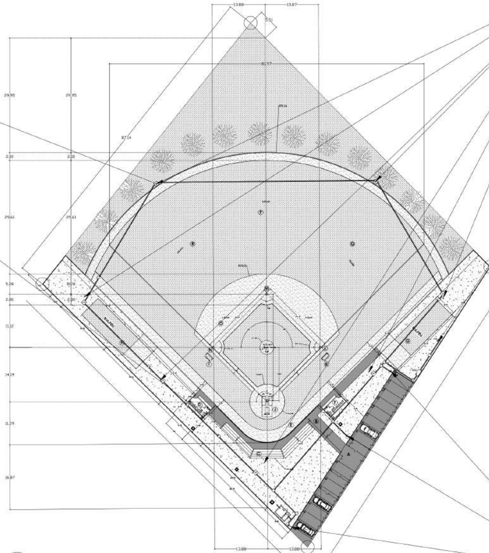
5 PLANTA ARQUITECTONICA DE CONJUNTO A-03 ESC: 1:300
