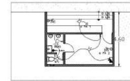
4 PLANO ELECTRICO A-04 DUGOUT ESC: 1:100
