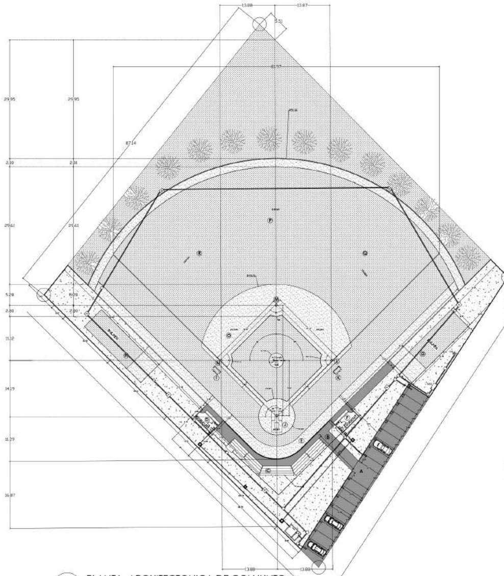
1 PLANTA ARQUITECTONICA DE CONJUNTO A-02 ESC: 1:300
