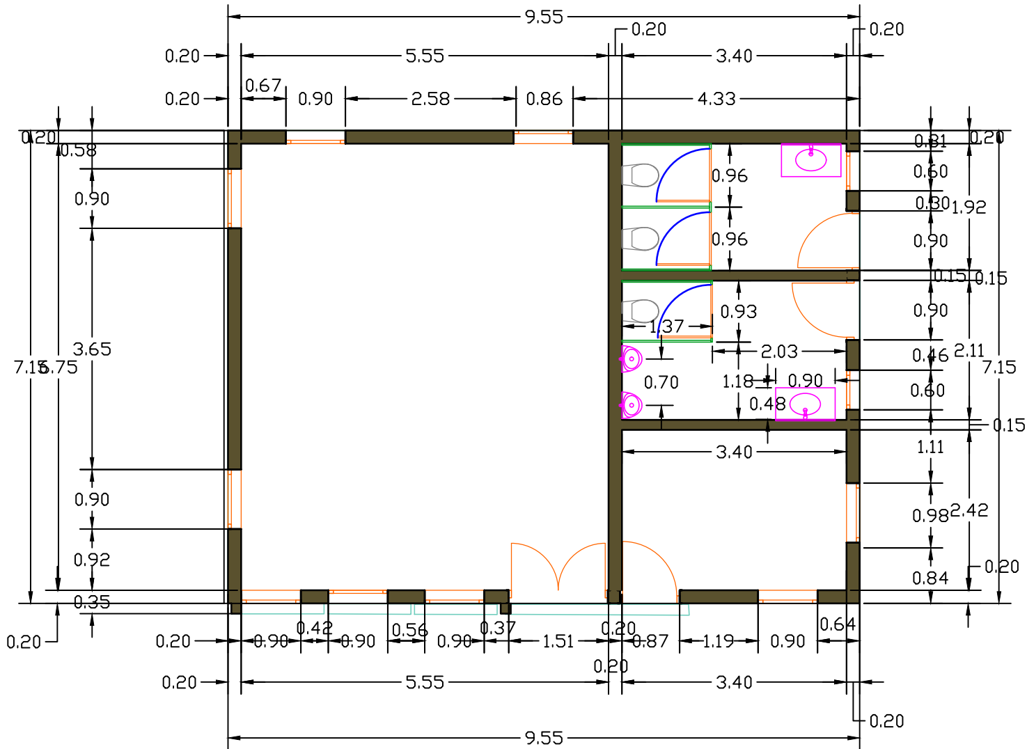
Planta Dimensionada
