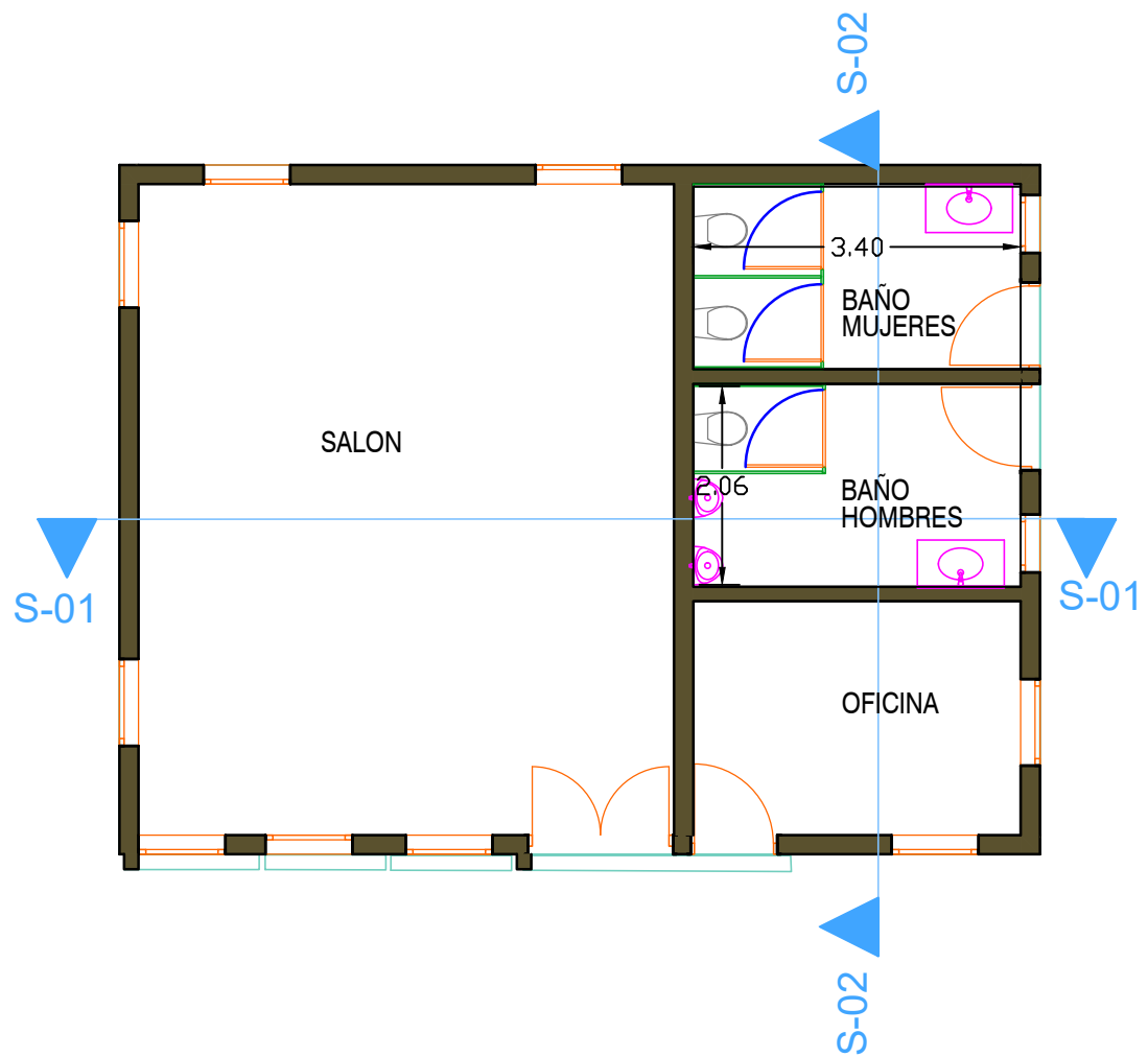
Planta Arquitectónica
